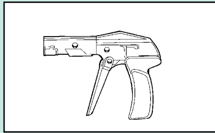
L-200 Stramme og kutteverktøy for buntebånd. Justerbar tiltrekingskraft før kutting. Max båndbredde 4,7 mm
